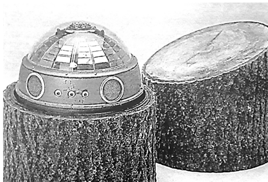
«Пенёк с начинкой» — радиоэлектронное устройство, установленное под Можайском.
