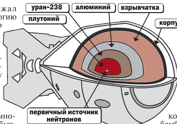
Схема «изделия» РДС-1 — первой советской атомной бомбы.
