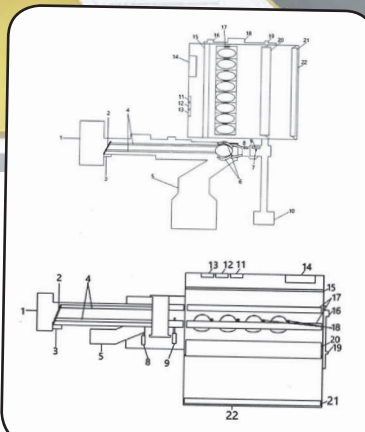
Так уникальный инкубатор выглядит на чертежах, его реальный вид пока держат в секрете.
